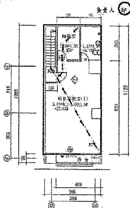
二樓變更後平面圖
